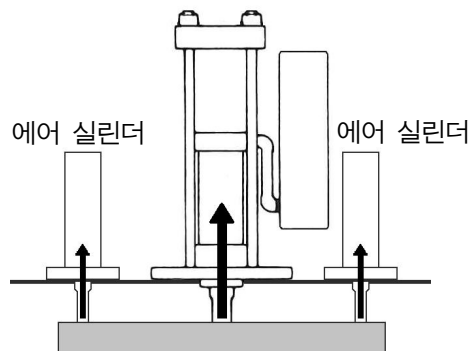
뉴매틱 파워 실린더
